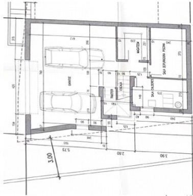
Planta garatge
