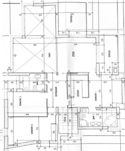
Planta dormitoris
