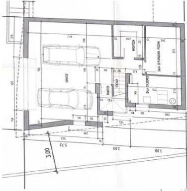
Planta garatge
